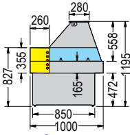
Oceanus gerades Frontglas
