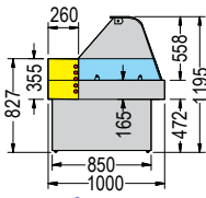
Oceanus gebogenes Frontglas
